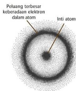
Teori Atom Mekanika Kuantum
