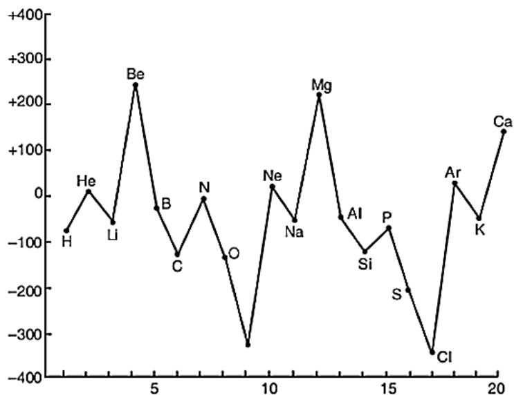
Grafik Energi Ionisasi
